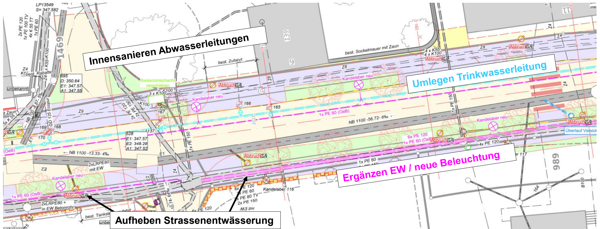
Werkleitungsplan Birrfeldstrasse, Porta AG
